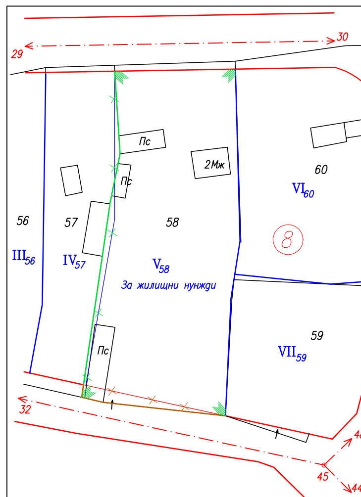
ЧИ на ПУП - ПЛАН ЗА РЕГУЛАЦИЯ М 1:1 000
