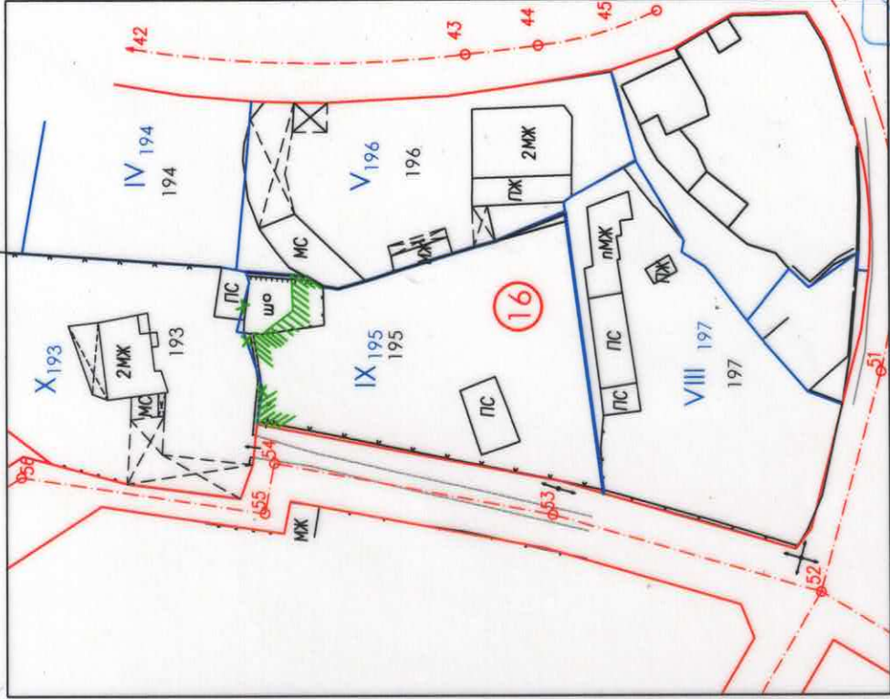
ЧИ НА ПУП - ПЛАН ЗА РЕГУЛАЦИЯ М 1:1 000
